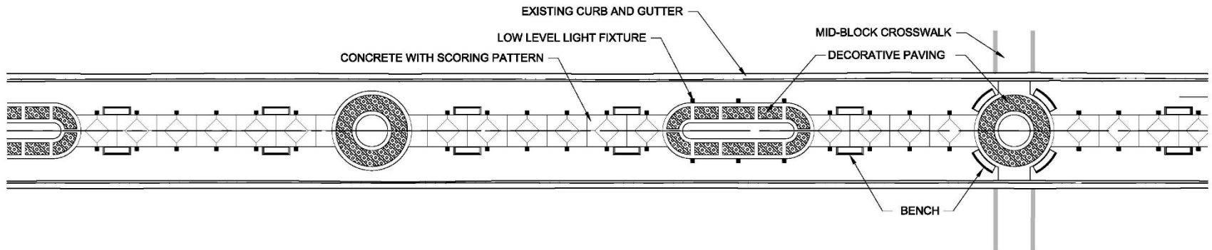
PROMENADE LAYOUT 'B'
