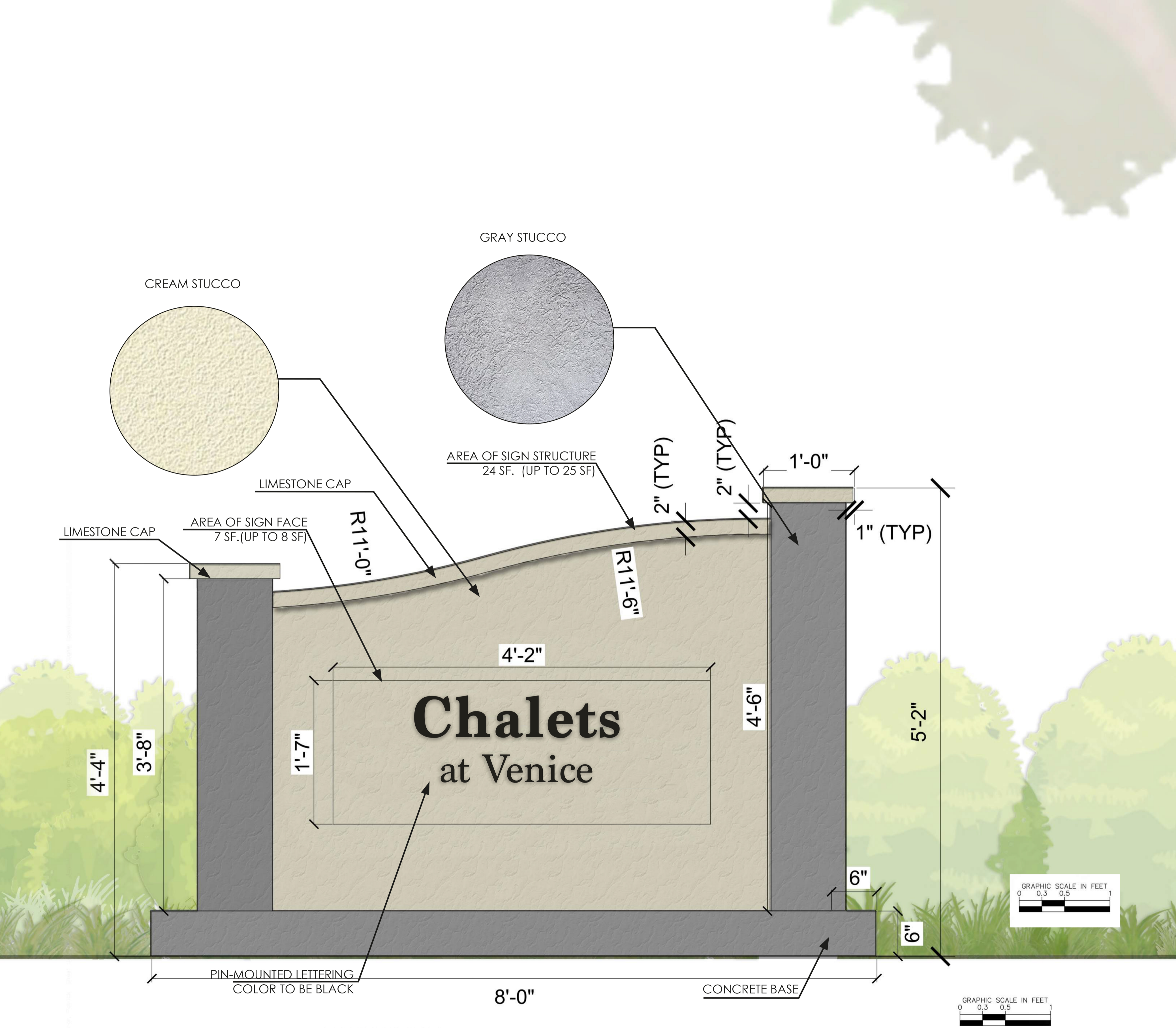
ELEVATION
